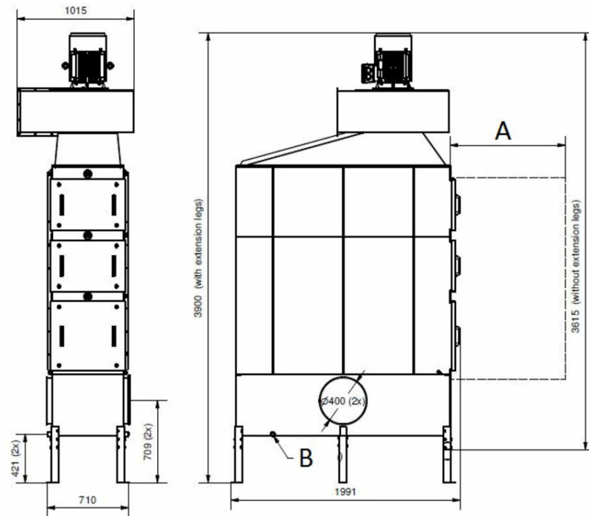
A) 1000mm维修空间 B) 排液口 DN25 (2x)
